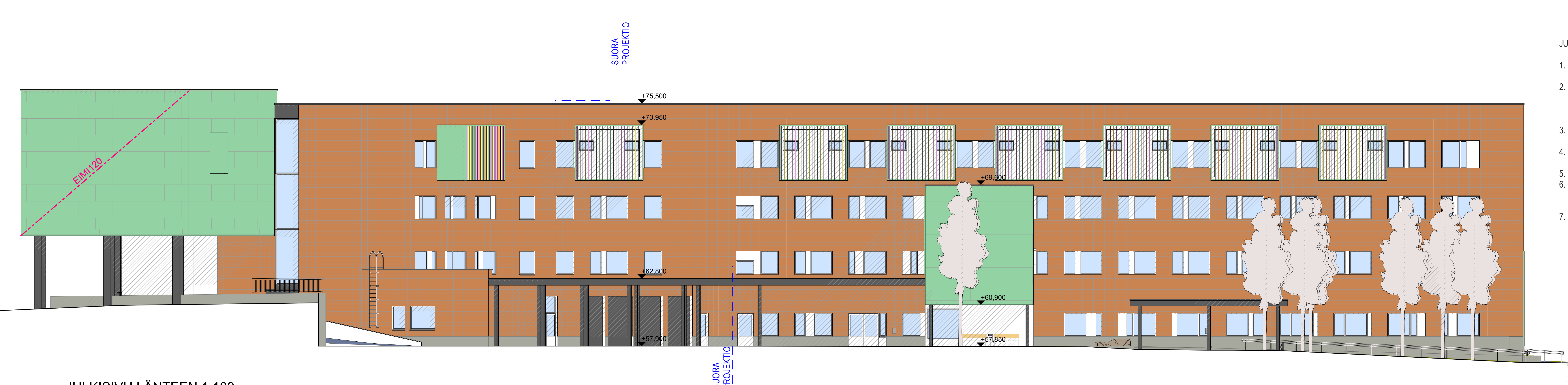
JULKISIVU LÄNTEEN 1:100
