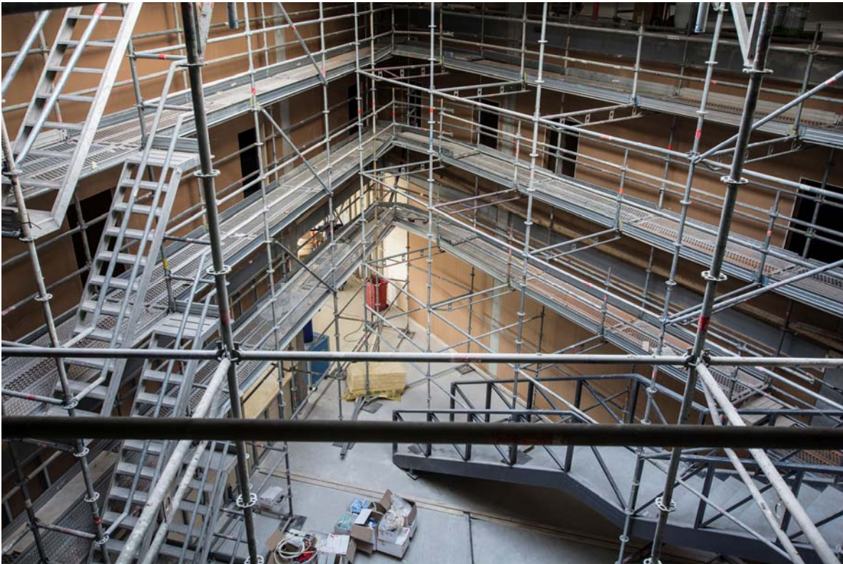
Seinätoitä varten pystytettyjä rakennustelineitä valokatteen alla olevissa tiloissa (kuva 3).
